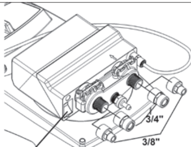
INGRESSO ADATTATORE (AC) ADAPTER INPUT
